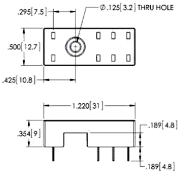
SC375-5.0
